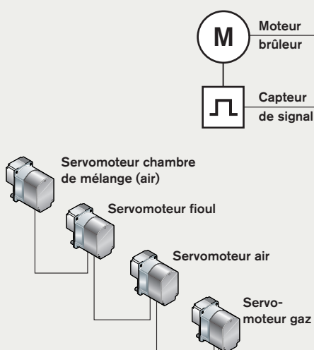
Brûleur avec manager de combustion numérique
