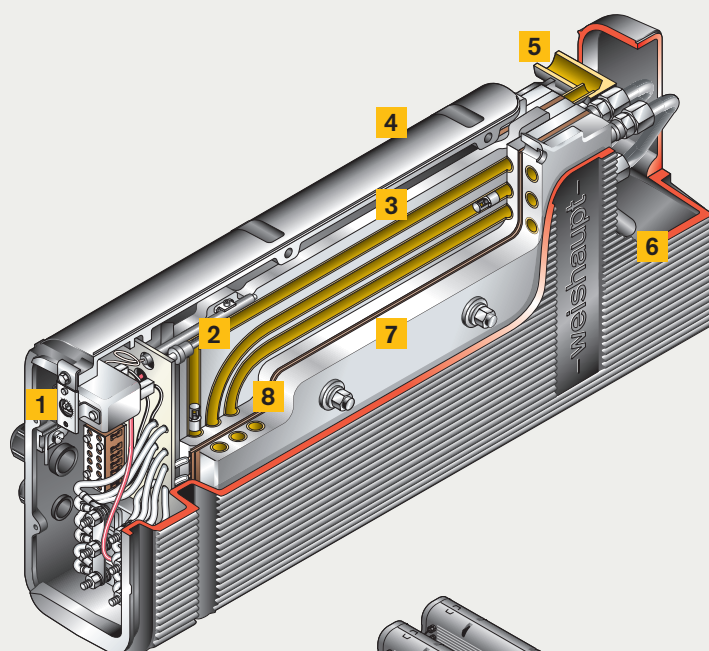
Réchauffeur électrique WEV2
