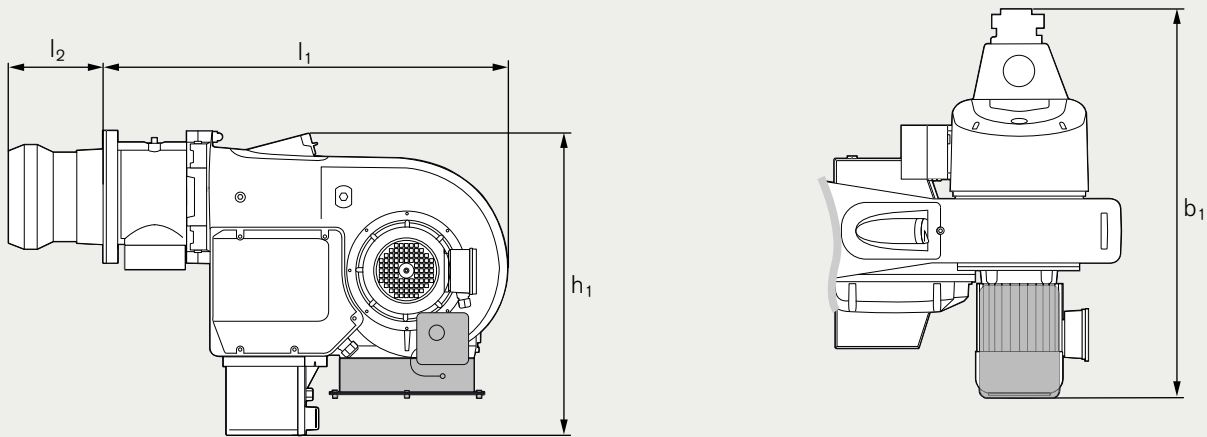
Dimensions - Exécution T / R / ZM-R
