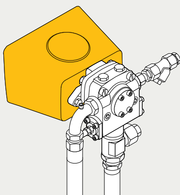
Accouplement magnétique pour brûleurs fioul dans le cas d'une ventilation permanente
