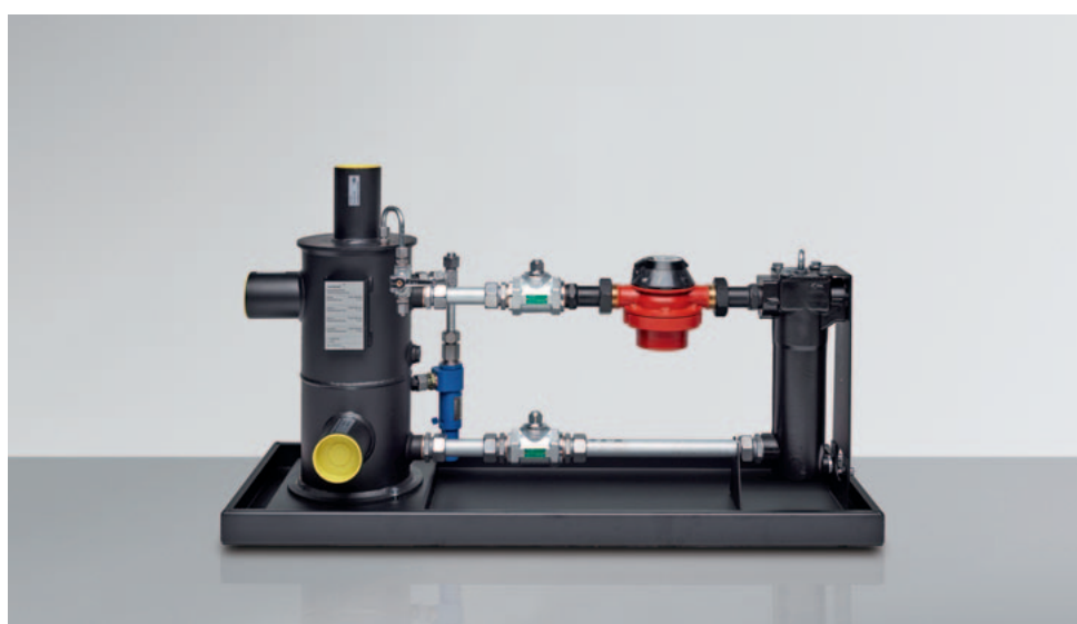
Pot de circulation avec volucompteur fioul
