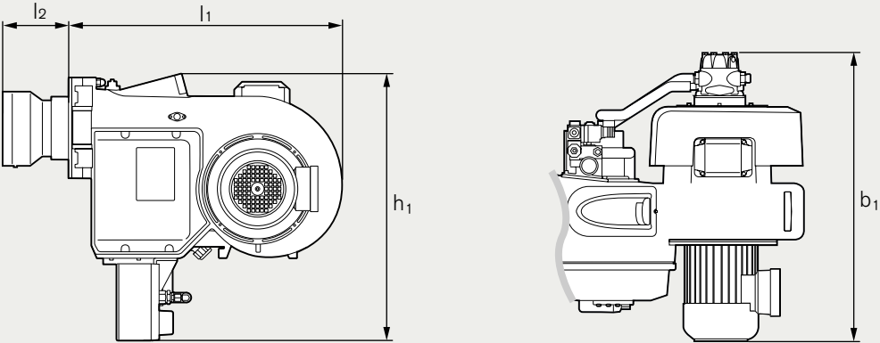
Dimensions - Exécution Z / T Réchauffeur fioul monté dessous (de série)
