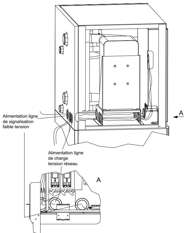
Fig. 7.3: Passage de câble du boîtier électrique
